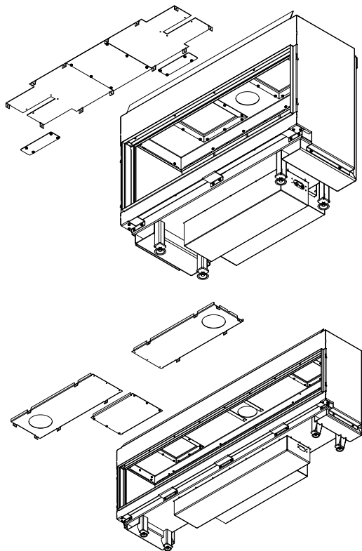
Rys. 13. Demontaż deflektorów LEO100 i LEO200
